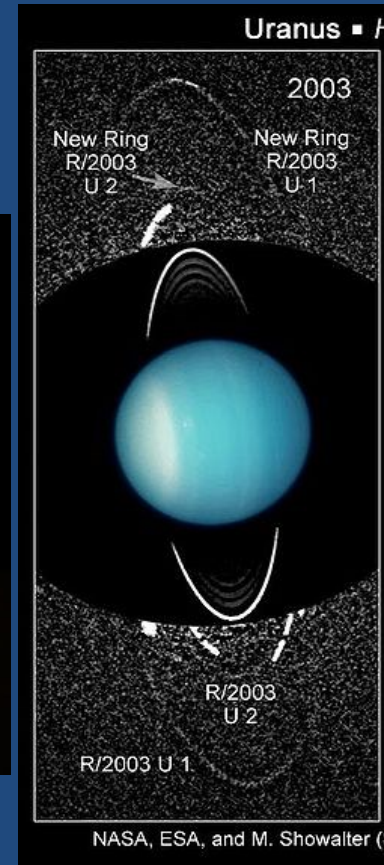
Uranus
